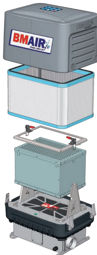
Kabiinikaitse MAO-3 aktiivsöe kombifilter
